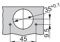
Kombinovani uzorak bušenja za impresso
