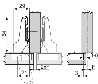
Polukoleno šarka
