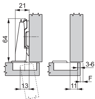
Ravna šarka
